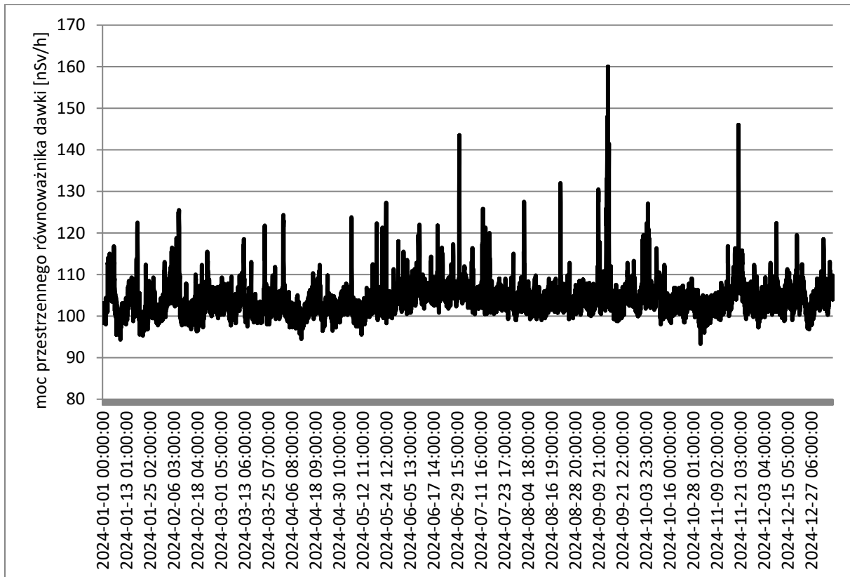
Rys. 2: Wyniki pomiarów mocy przestrzennego równoważnika dawki w 2024 roku.
